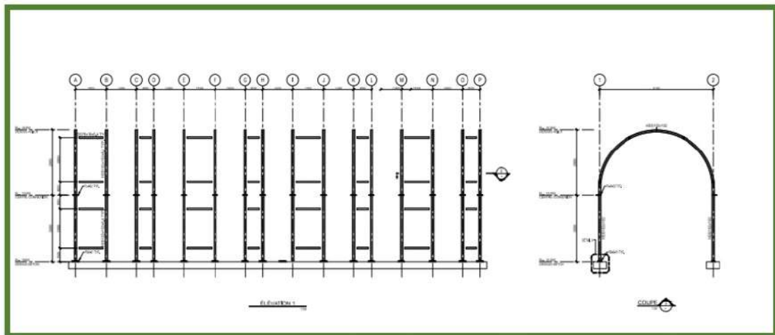
Carte 5. Dessins de la structure portante interne des arches.
